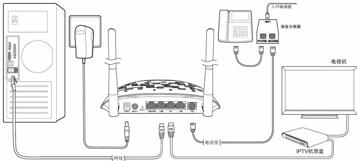
图 3 ADSL 宽带
