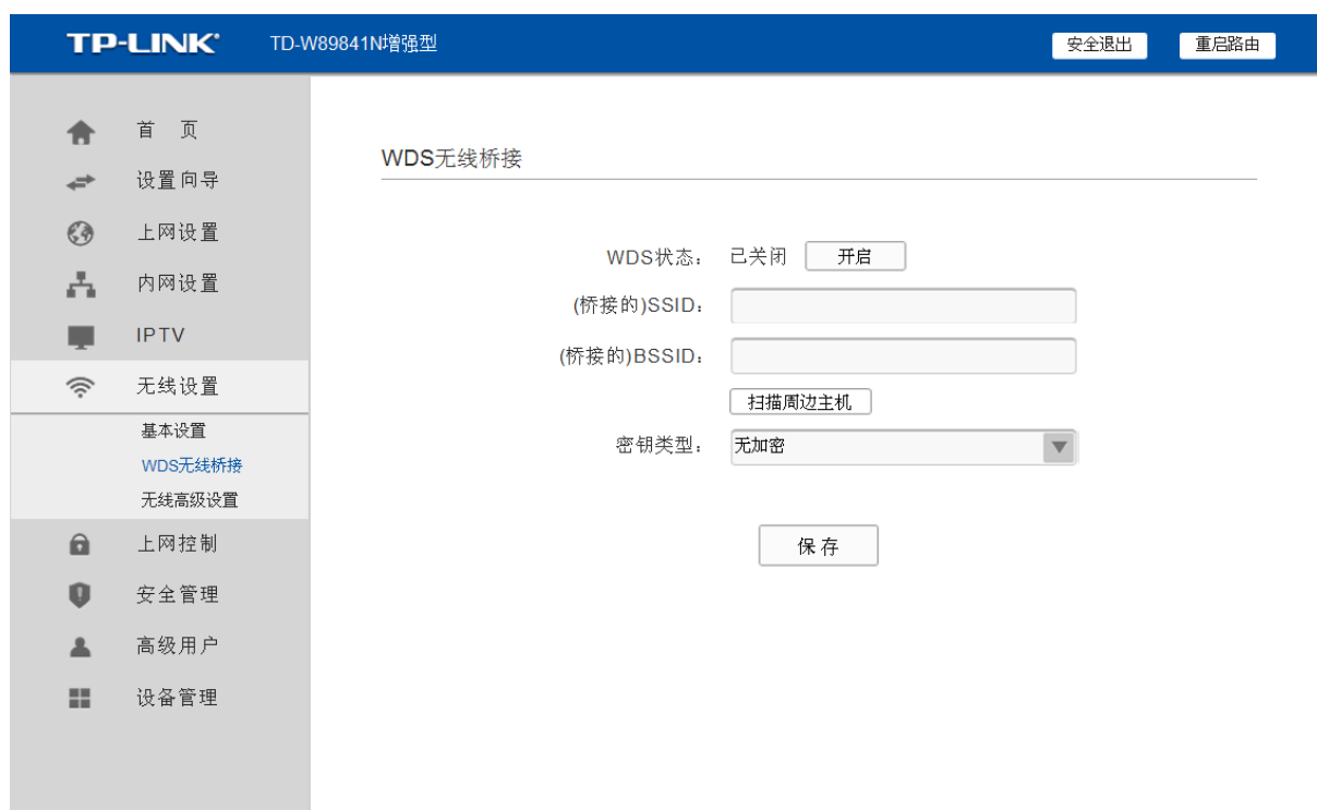
图 43 WDS 无线桥接
