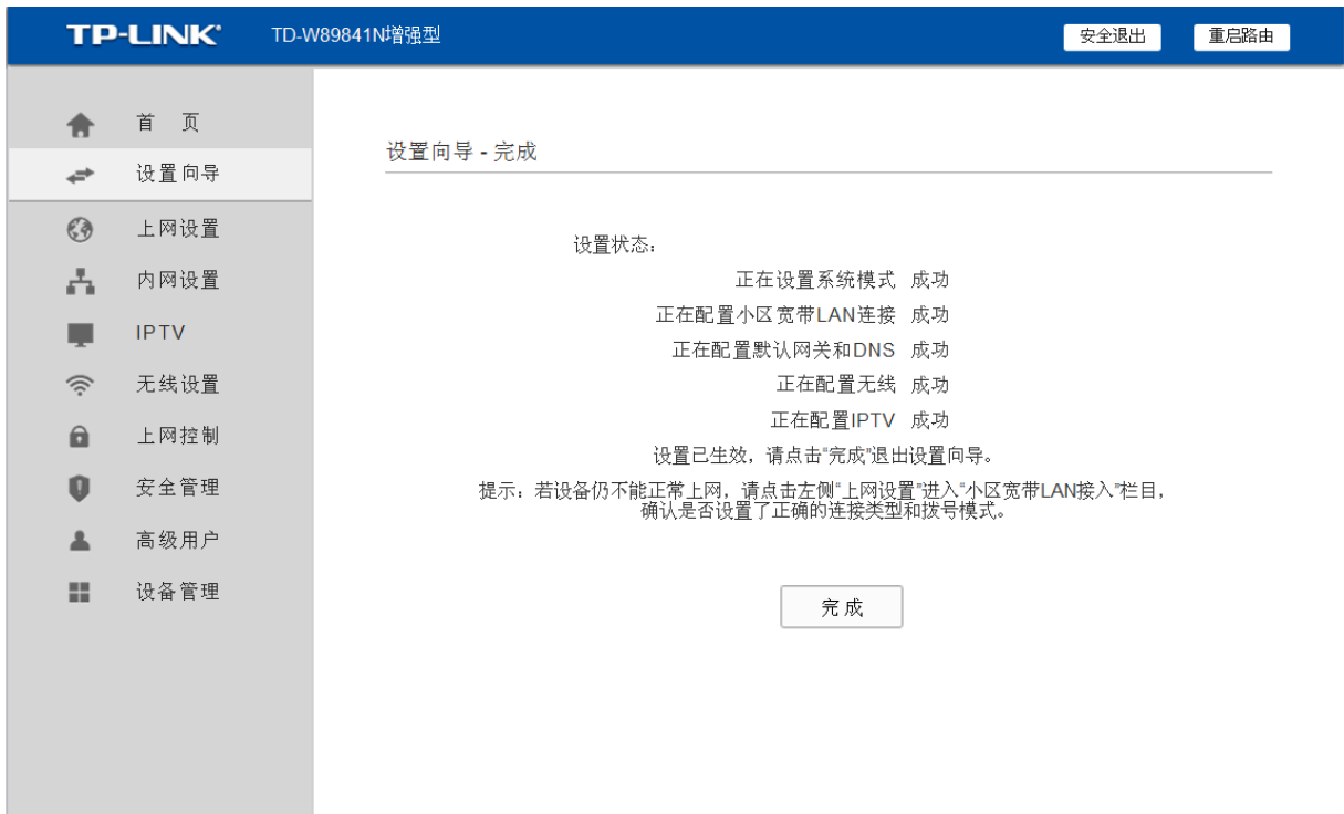
图 21 设置向导一完成
