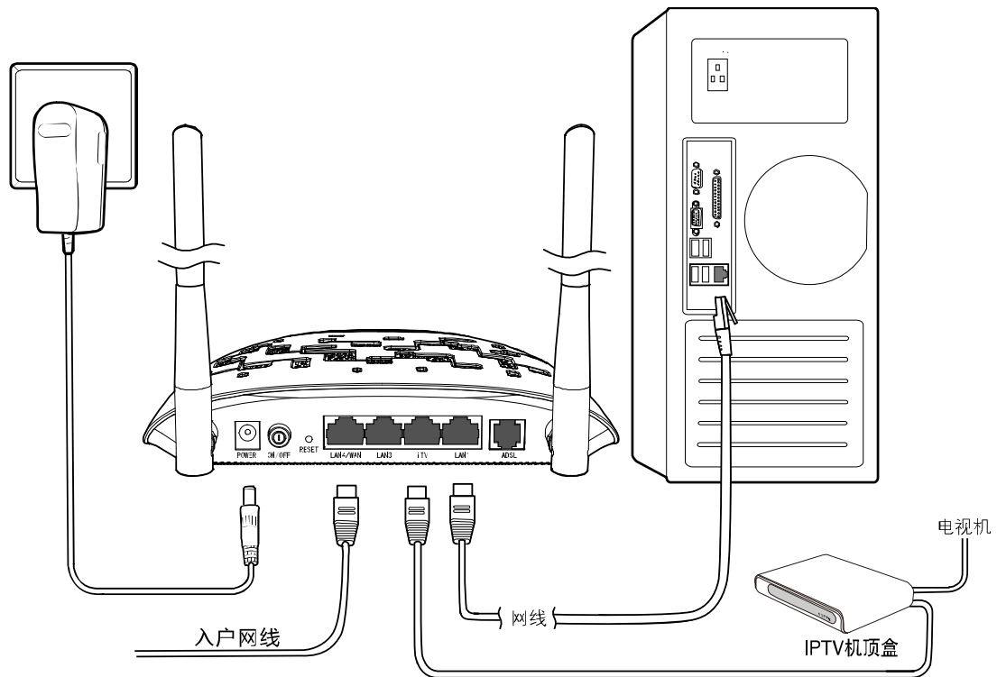
图 4 小区宽带
