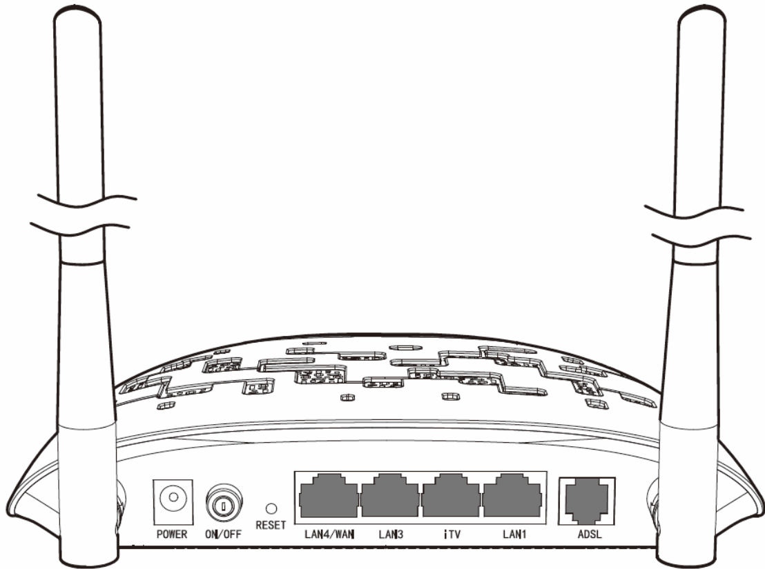
图 2 TD-W89841N 后面板示意图
